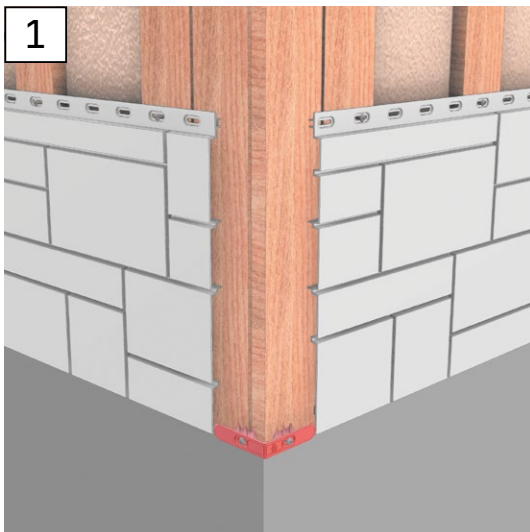
Рис. 19 Монтаж первого ряда панелей
