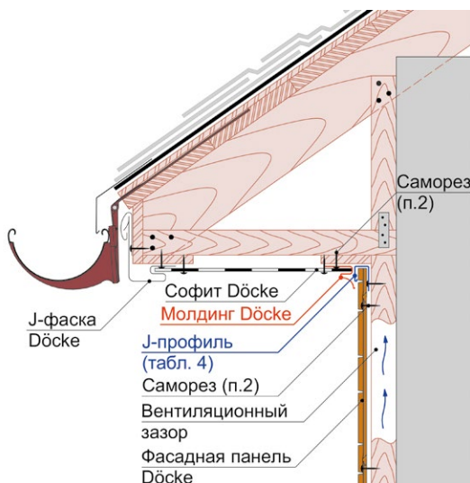
Рис. 22 Примыкание фасадных панелей Döcke к карнизному свесу.
