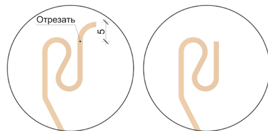
Рис. 10 Подрезка стартового профиля для сайдинга под дерево.
