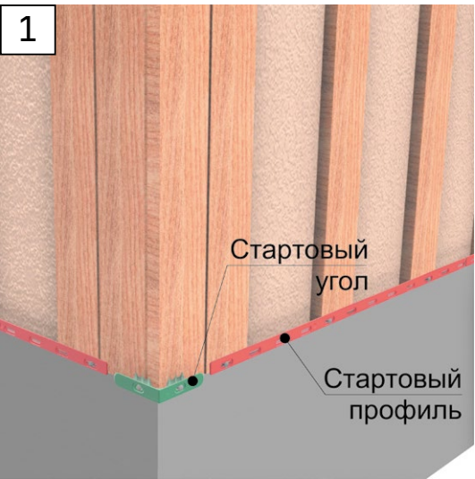
Рис. 9 Установка стартовых профилей и стартовых углов
