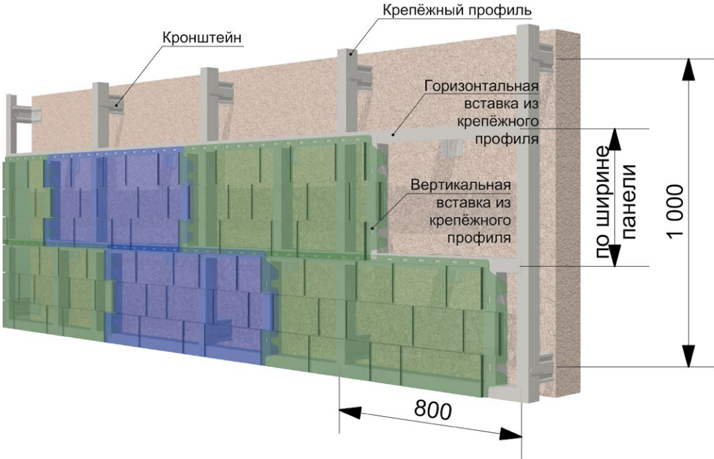
Рис. 8 Установка вертикальных вставок
