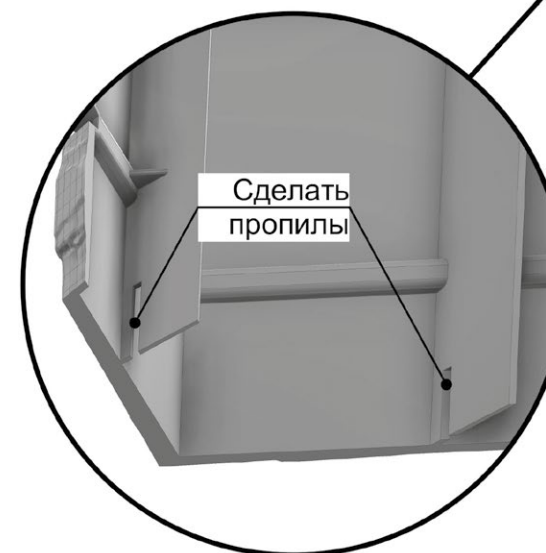
Рис. 21 Отделка цоколя с перепадом высоты
