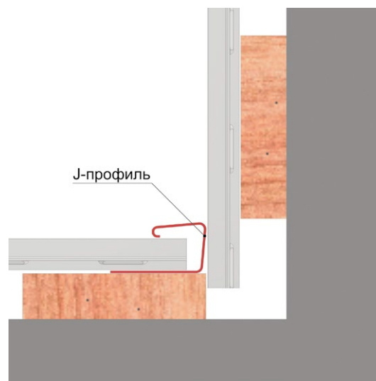
Рис. 16 Монтаж обрешётки под внутренний угол
