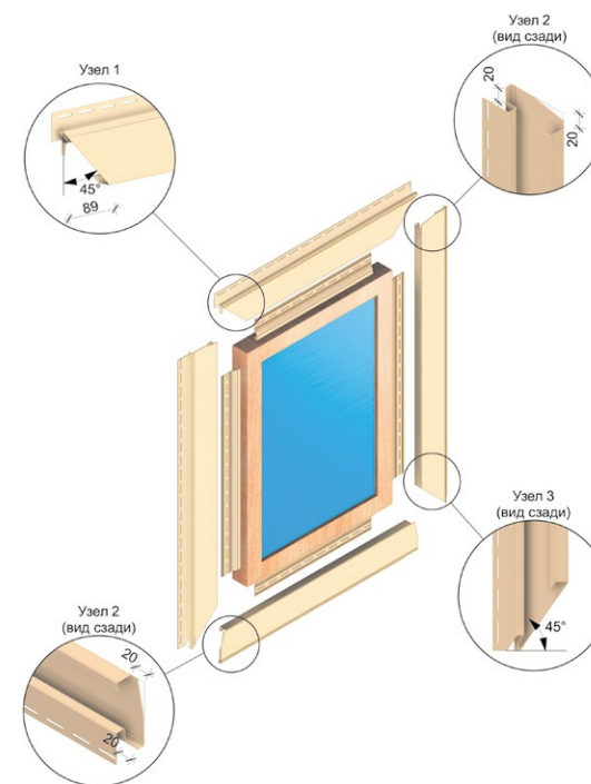
Рис. 11 Обрамление оконного проёма при помощи наличника 89/30 мм.
