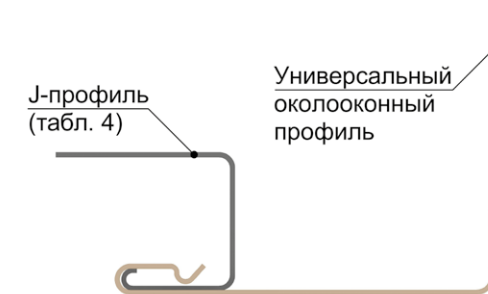
Рис. 12 Соединение универсального околооконного профиля с соответствующим J-профилем (таблица 4).
