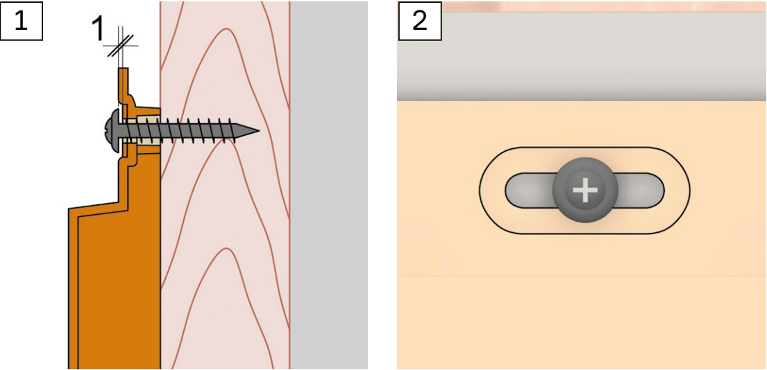
Рис. 2 Схема фиксации фасадных панелей Döcke
