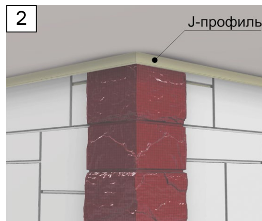
Рис. 24 Примыкание внешнего угла Döcke к карнизному свесу.
