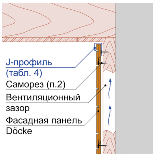
Рис. 23 Примыкание фасадных панелей Döcke к горизонтальной поверхности
