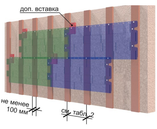
Рис. 6 Вертикальная обрешётка под фасадные панели Döcke STEIN и АЛТАЙ
