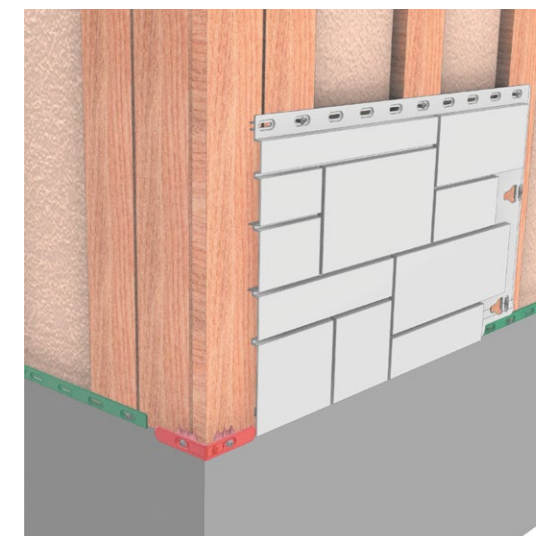
Рис. 18 Монтаж первой панели
