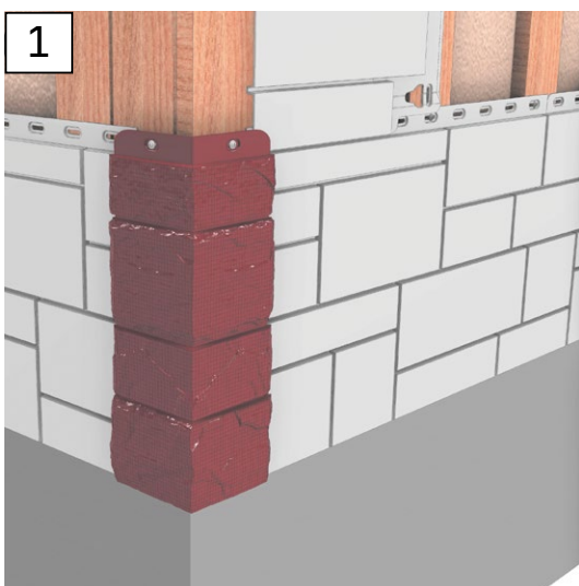
Рис. 20 Монтаж последующих рядов панелей
